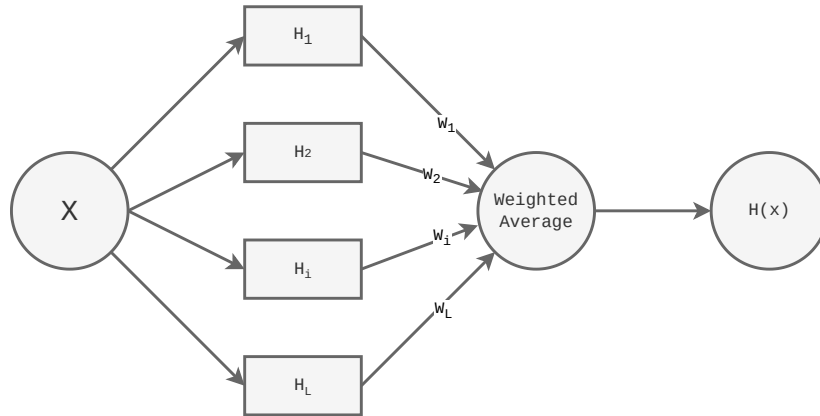
Figura 10.2: Esempio di ensemble learning tramite weighted averaging: ogni modello H_i ha un peso associato w_i che riflette la sua affidabilità. La previsione finale H(x) è una media pesata delle previsioni dei modelli base.
