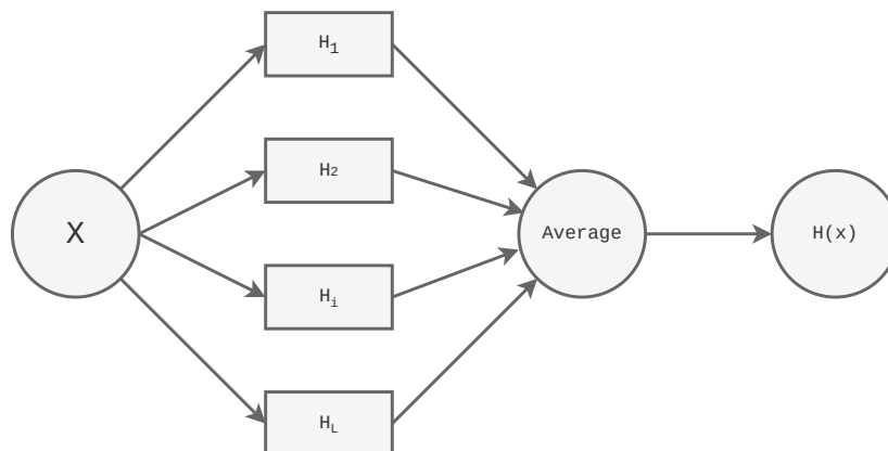
Figura 10.1: Esempio di ensemble learning tramite averaging: esistono L modelli H_1, H_2, \dots, H_L che fanno previsioni su un dato input x . La previsione finale H(x) è la media delle previsioni dei modelli base.
